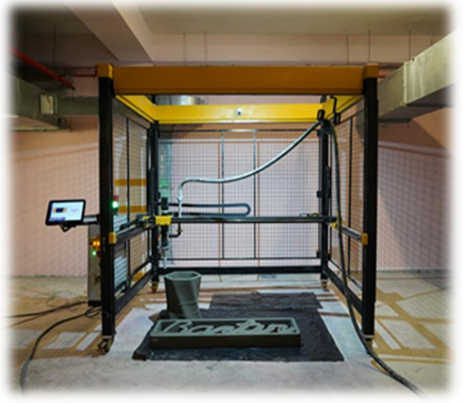
3D Beton Yazıcı
